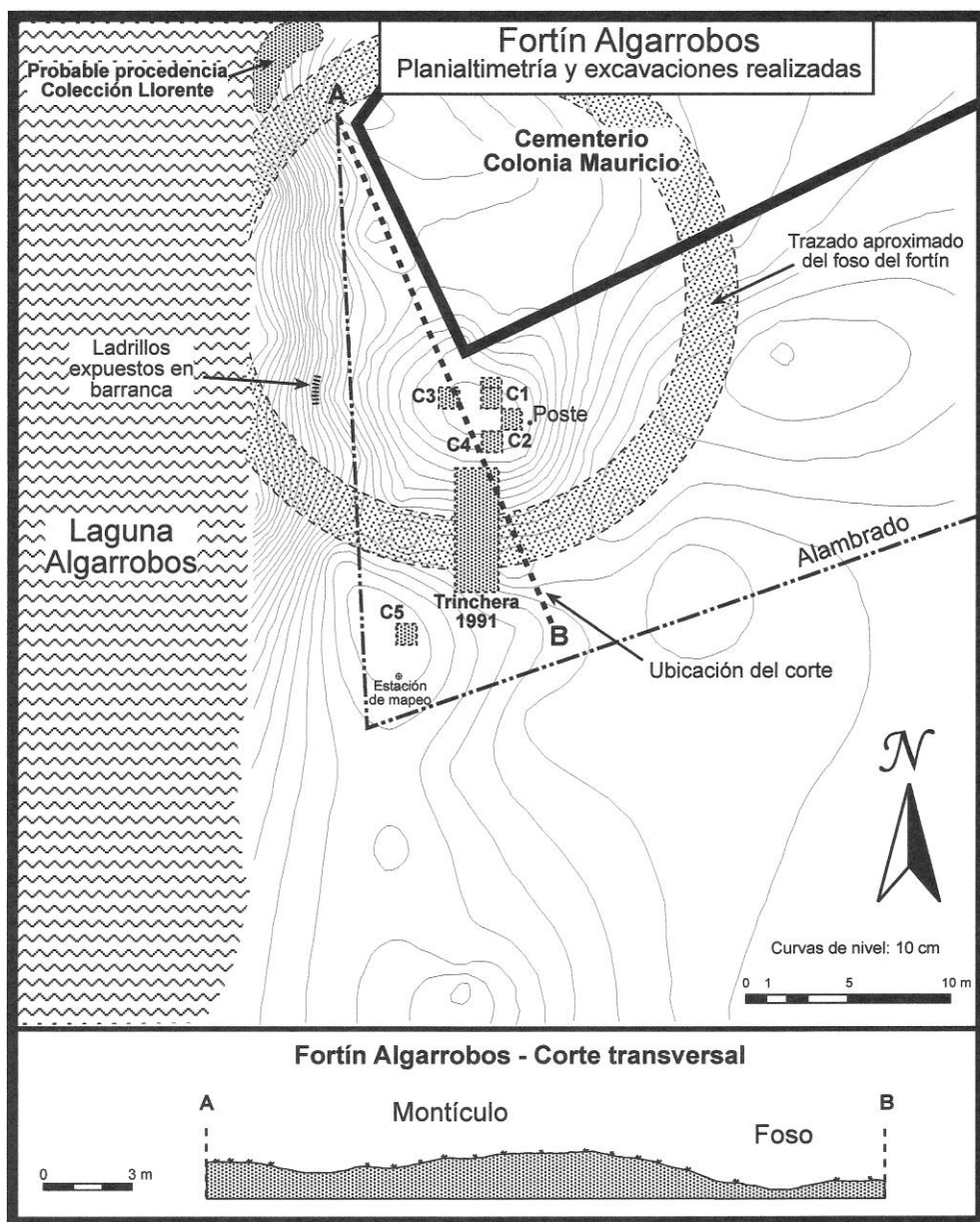
Figura 3. Planialtimetría y corte topográfico longitudinal del sitio Fortín Algarrobos, indicando la ubicación de las cuadrículas excavadas
