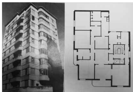
Figura 7. Edificio Arijón. San Lorenzo 1501 y Paraguay 610-20 (Rosario). Arqs. H. Larguía y Newton, 1933-34. Fuente: VV. AA., Hilarión Hernández Larguía
