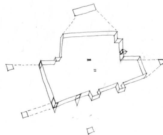
Figura 107b. Croquis conceptual de la perforación del muro que encorseta la planta fija a través de abrir ventanas en puntos estratégicos detectados. Elaboración propia.
