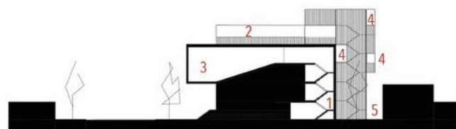
CORTE A-A
