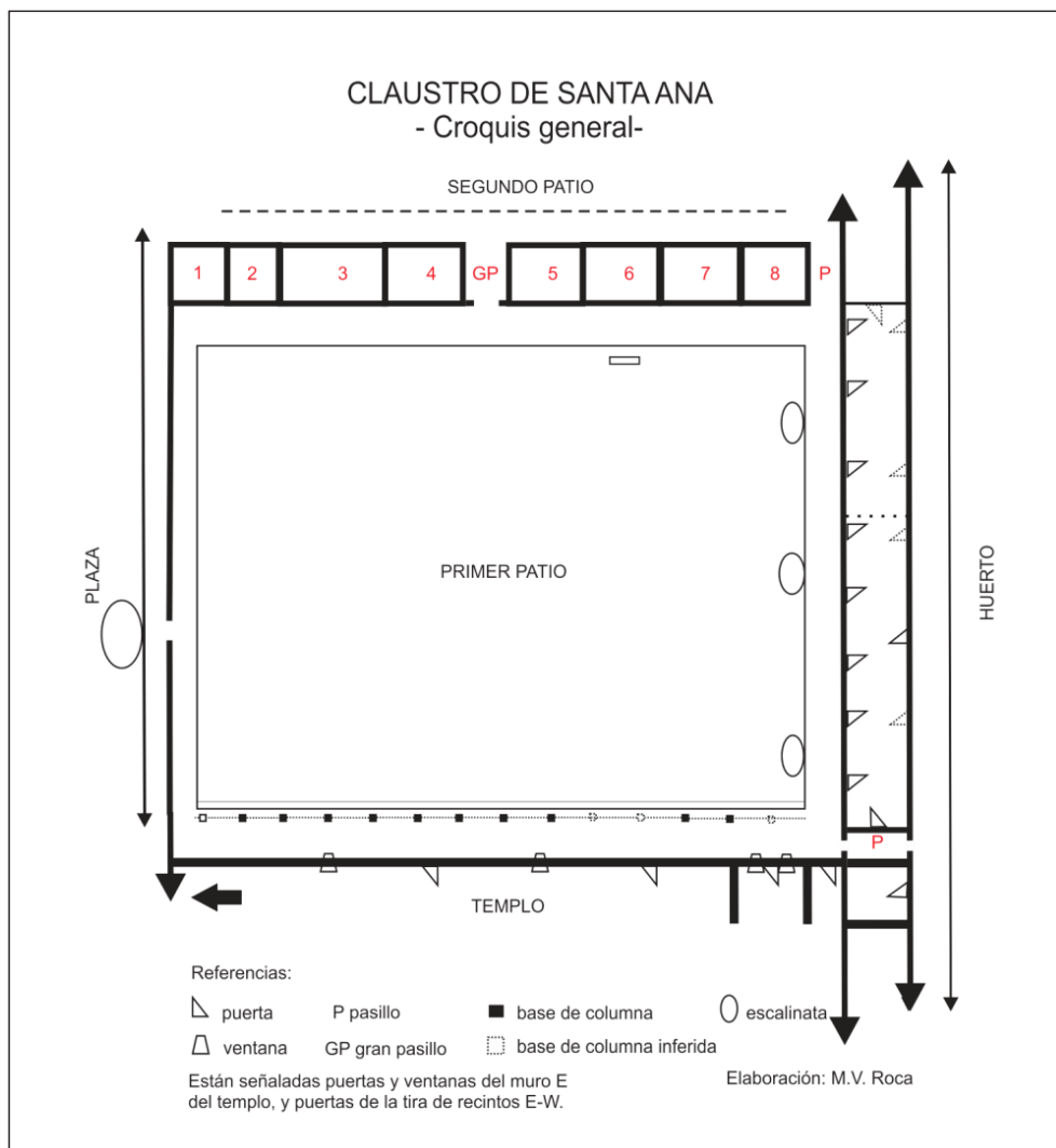
Figura 3: Croquis del claustro de Santa Ana. Elaborado a partir de planos existentes, análisis de fuentes documentales y datos de los recientes trabajos de campo. Fuente. Elaboración propia.
